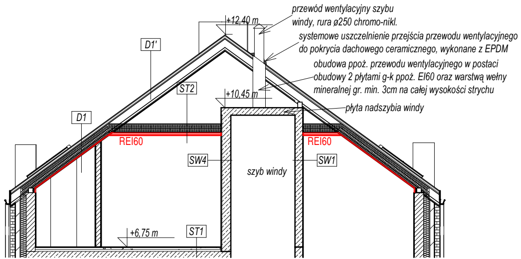
1 | Przekrój - went. windy 1 : 100
