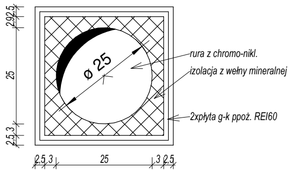
2 | Detal - obudowa went. szybu 1 : 10
